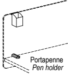
L. 60 / 80 / 100 / 110 / 120 / 130 / 160 / 180 H. 48 cm.
